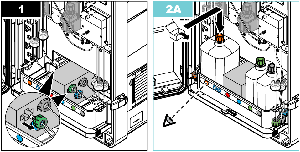
图 14 化学品安装
