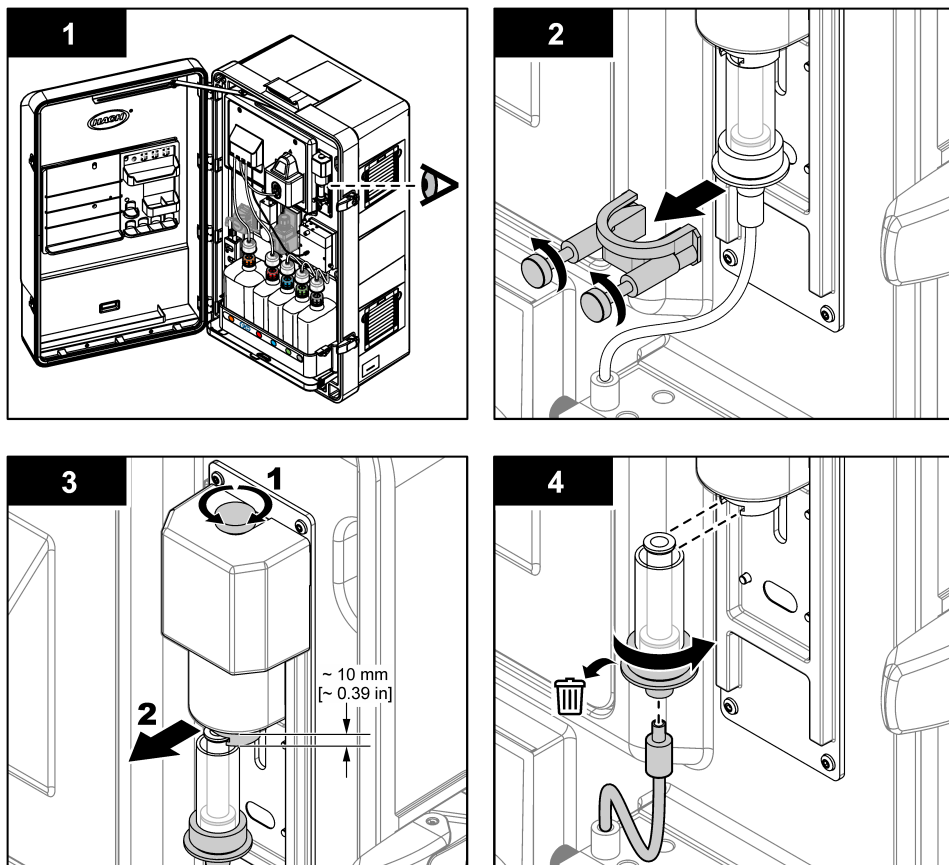
图 18 活塞泵更换
