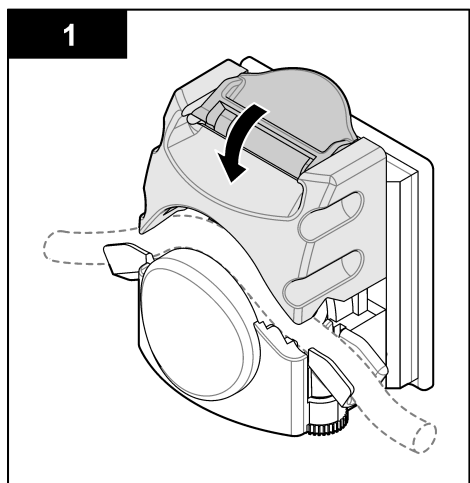
图 10 关闭夹杆
